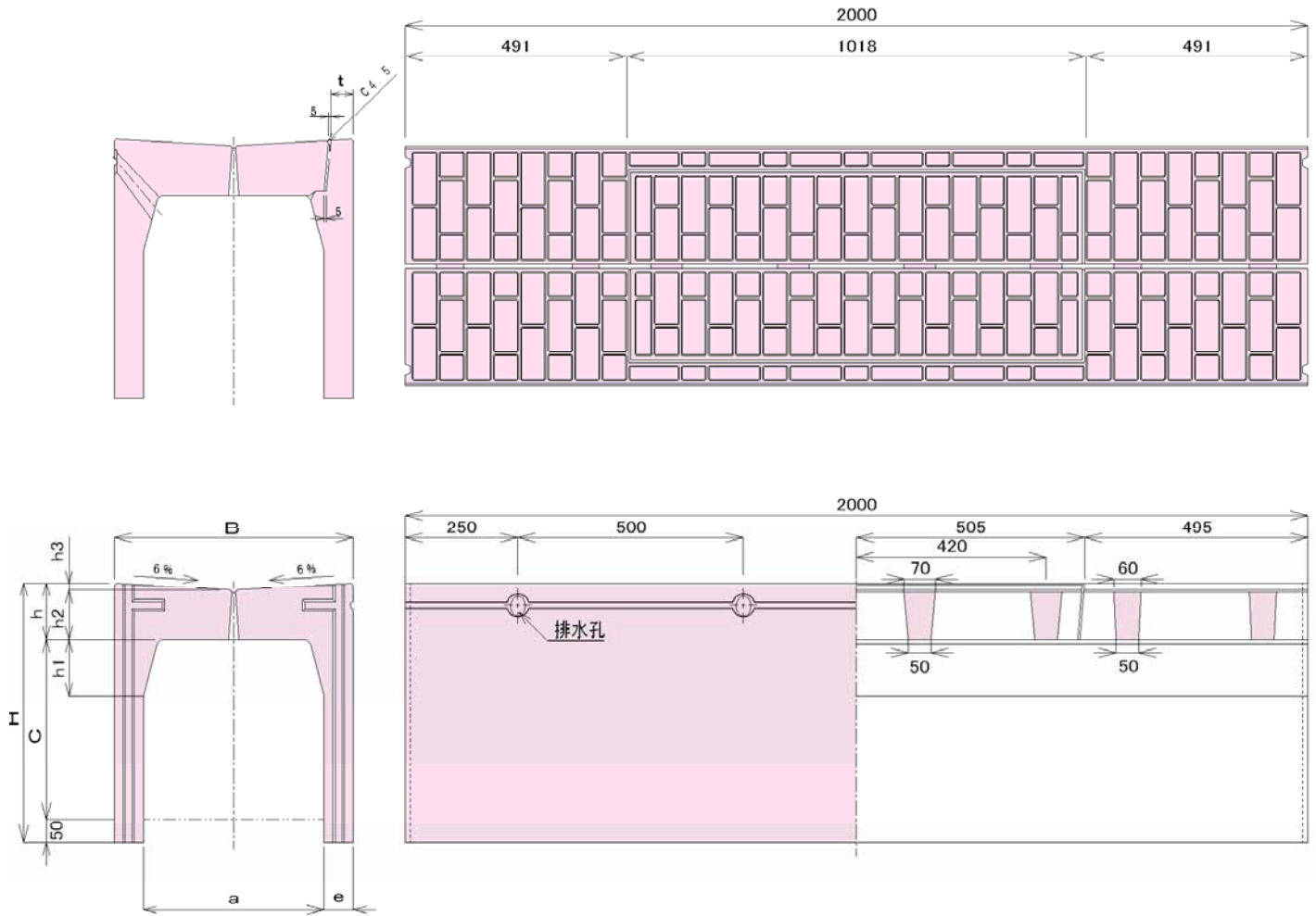
都市型可変側溝 (Cドレーン) T-25
